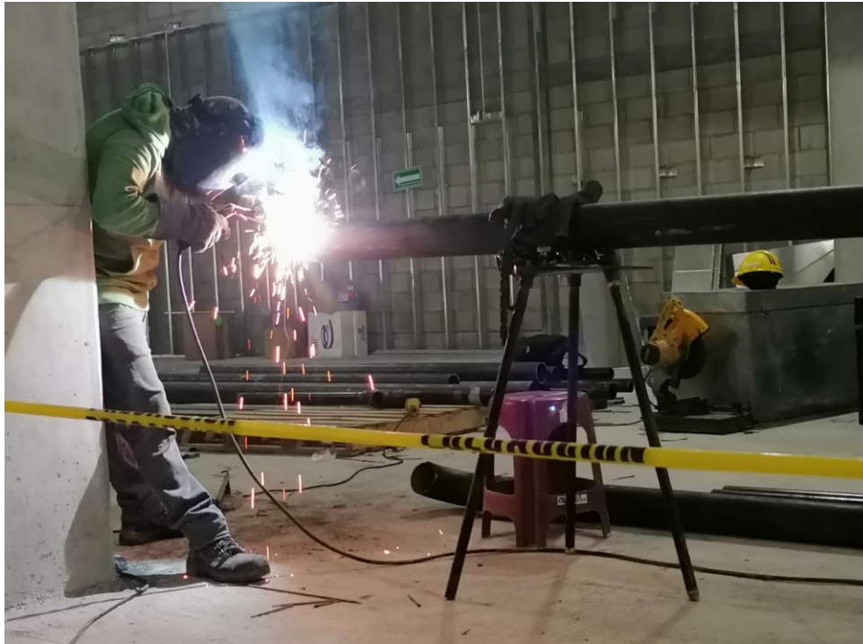
Trabajos de corte y soldadura.
